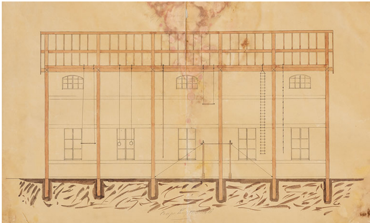
Projet de gymnase, coupe longitudinale.
