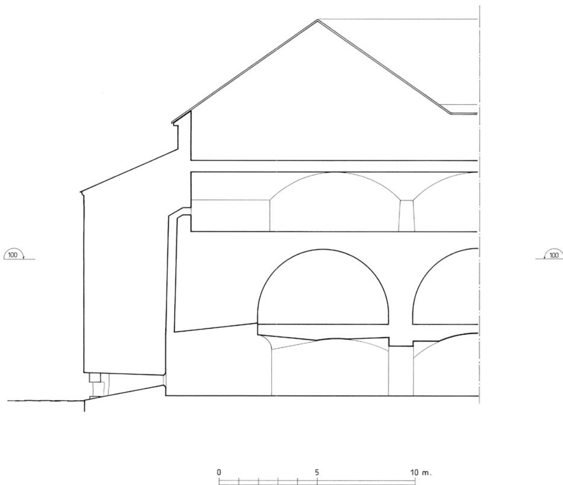
COUPE C - C'
