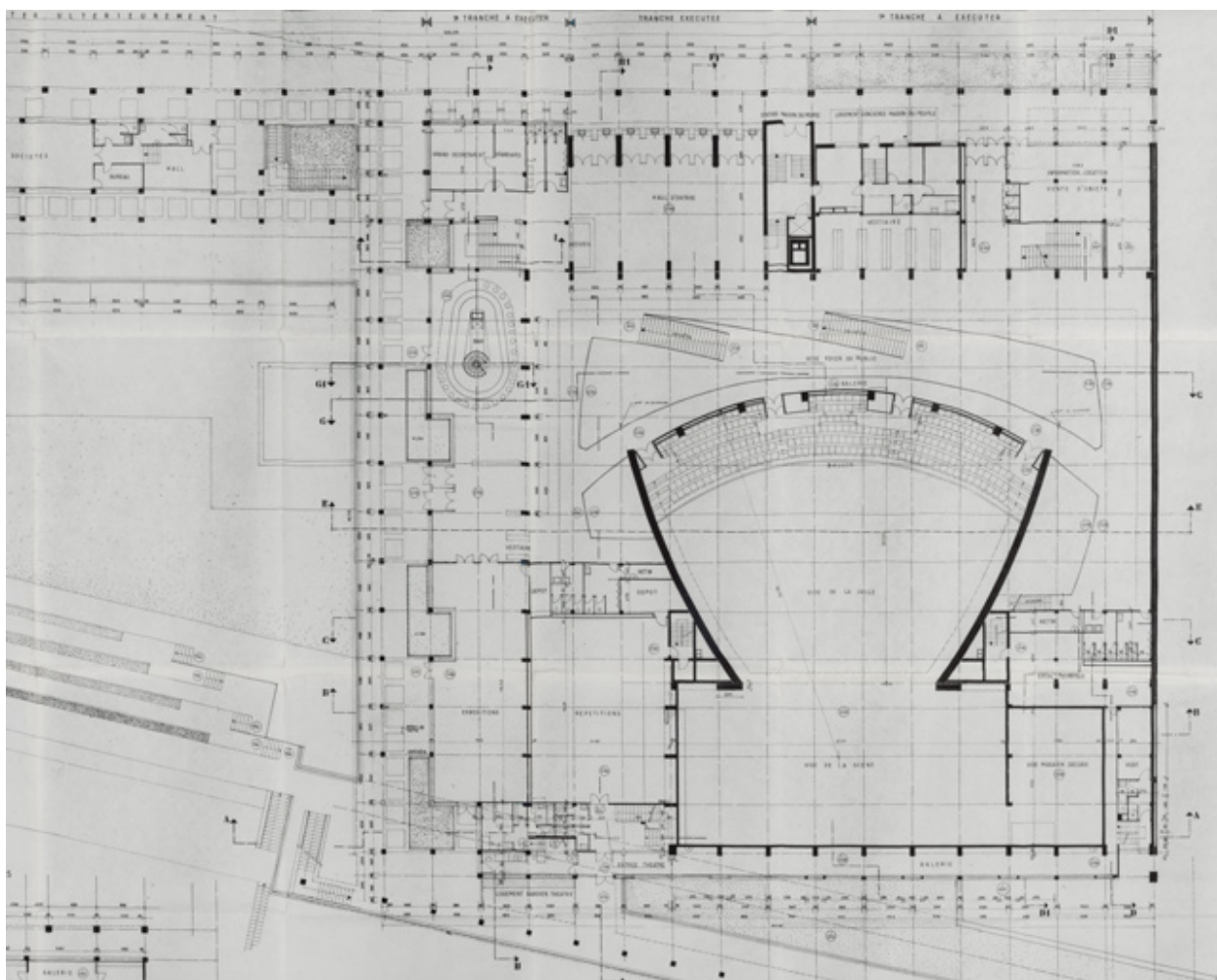
Nevers Centre municipal. Maison de la culture. 7. Plan d'exécution. Niveau rue, hall d'entrée [... Détail : partie droite]. Octobre 1964, rect. novembre 1964.
