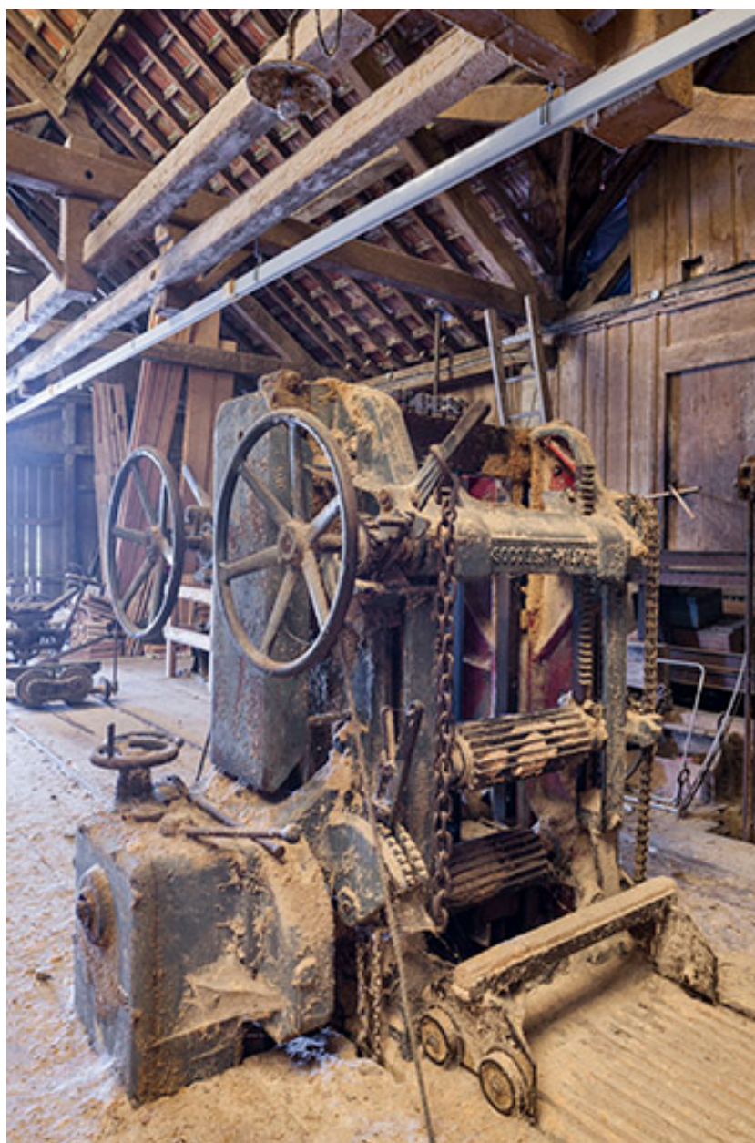
Châssis multilames vu de trois quarts arrière.
