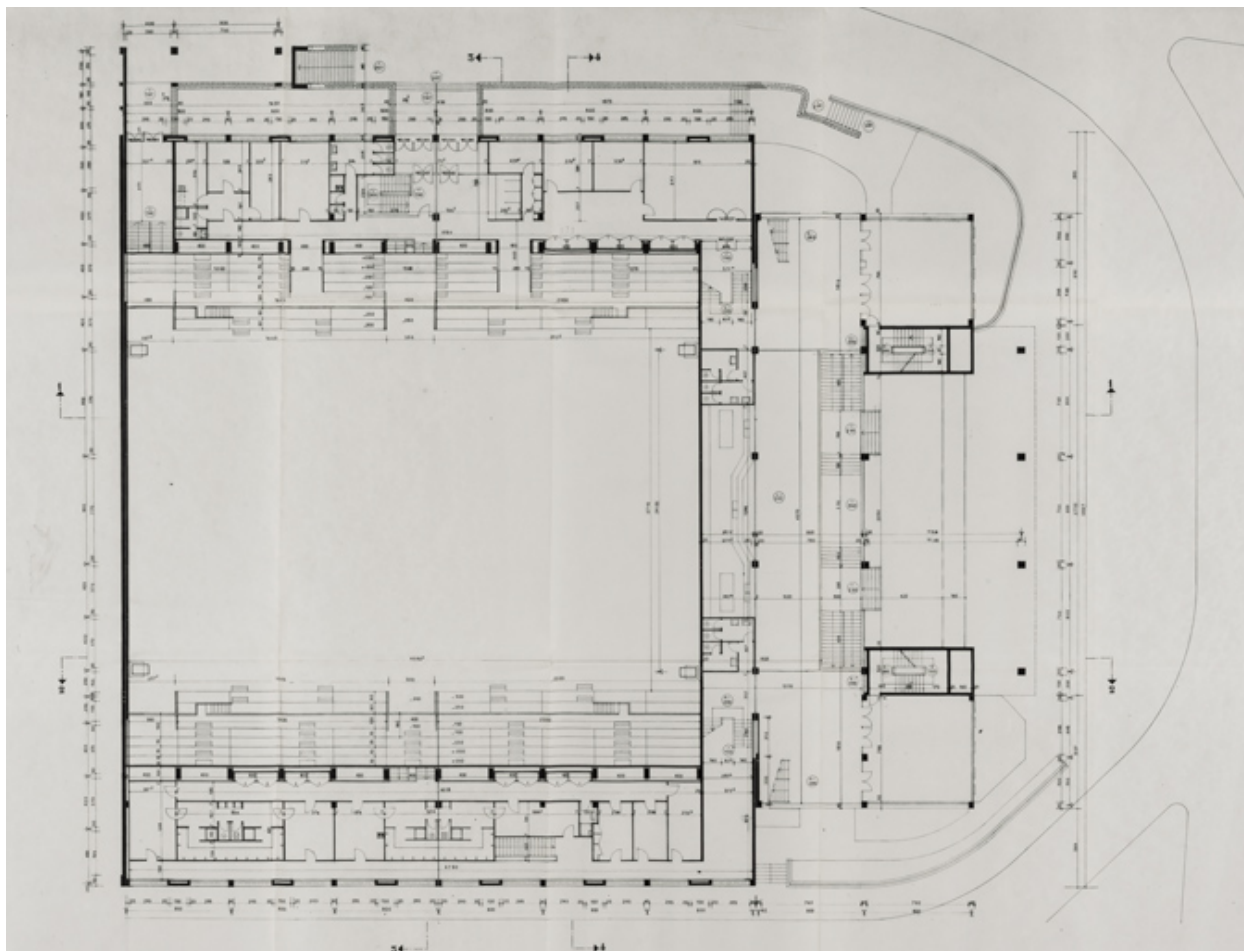
Nevers Centre municipal. Maison des sports. 6. Plan d'exécution. Niveau -150. Octobre 1964.
