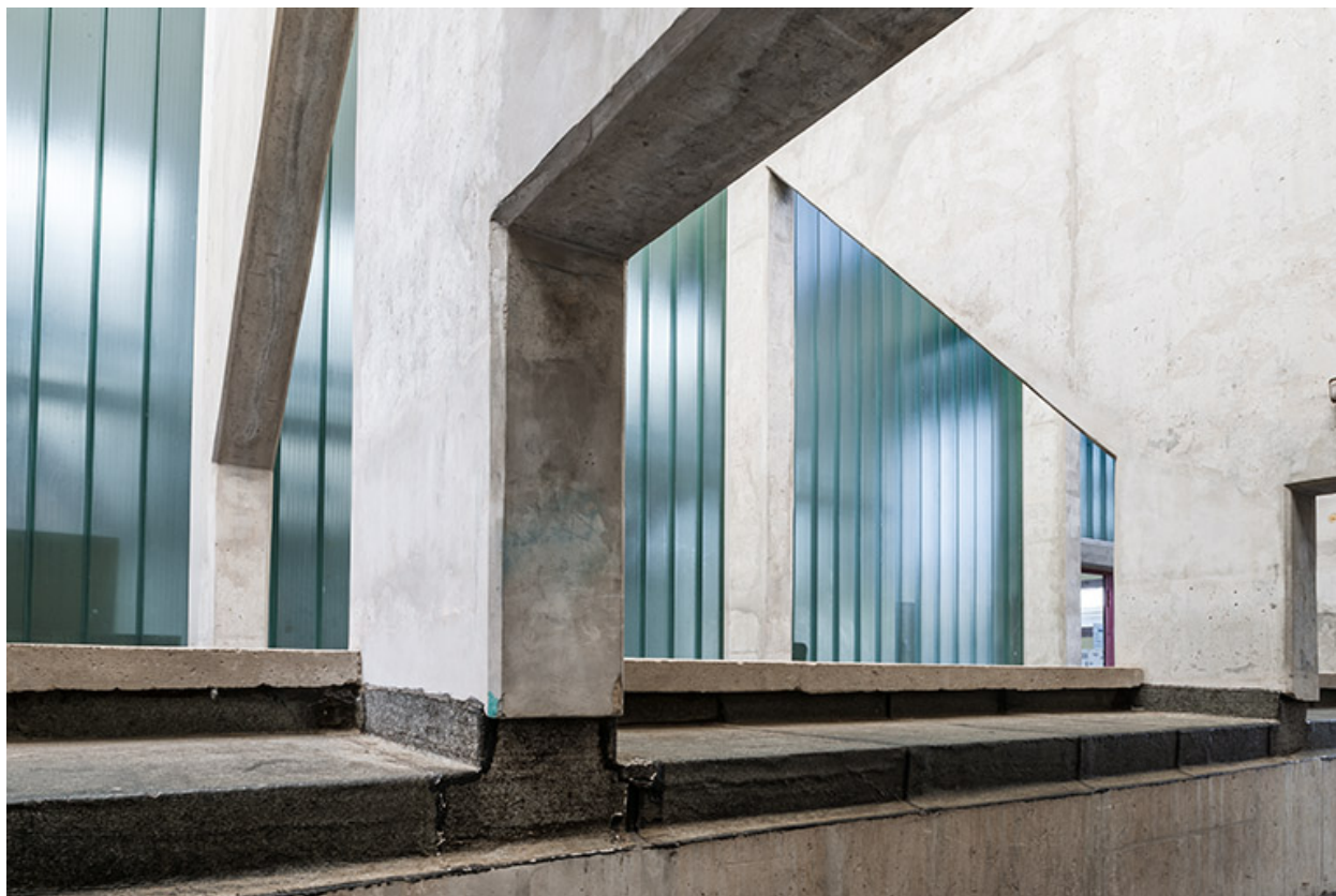
Atelier : détail ossature béton
