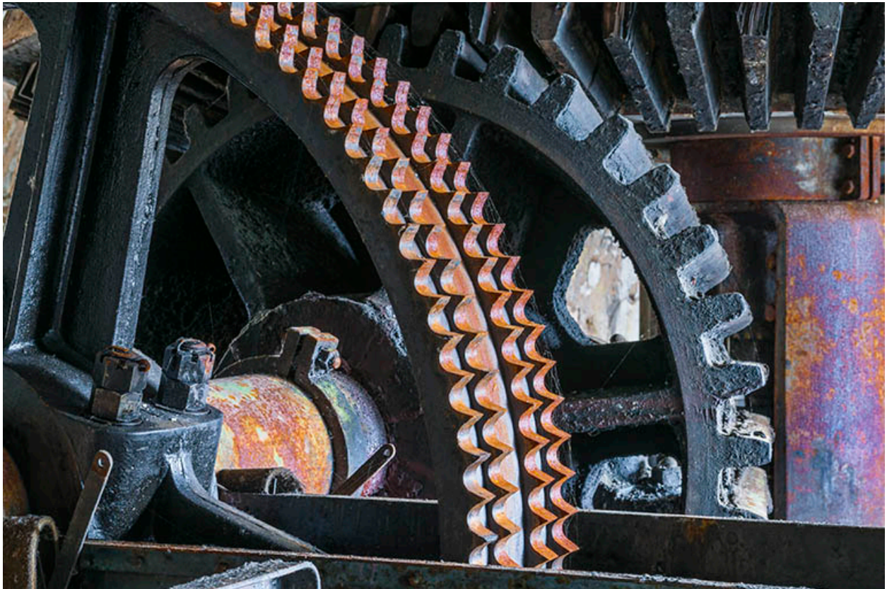
Rez-de-chaussée de l'atelier principal. Détail du mécanisme d'entraînement (engrenages coniques et roues dentées pour chaînes).
