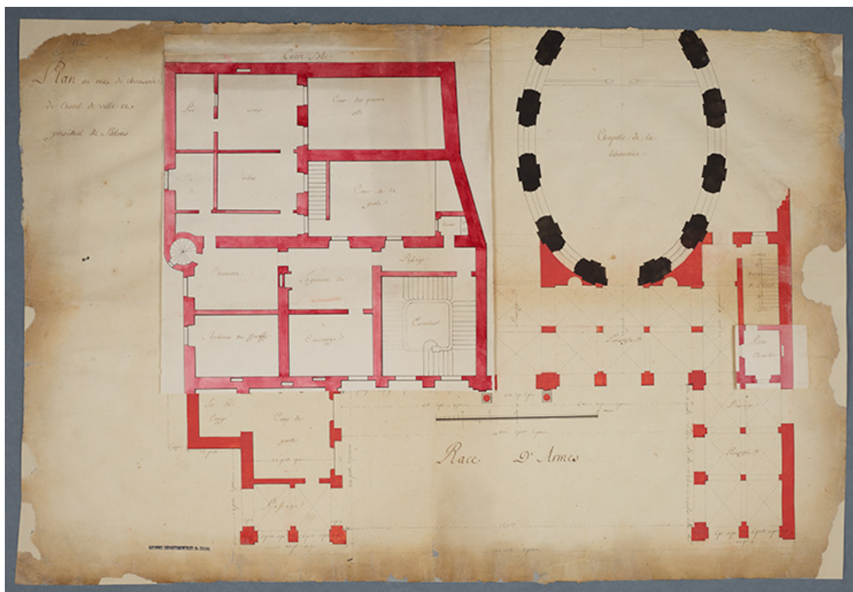
Plan du rez de chaussée de l'hotel de ville et présidial de Salins (avec entresol), s.d. [vers 1720].
