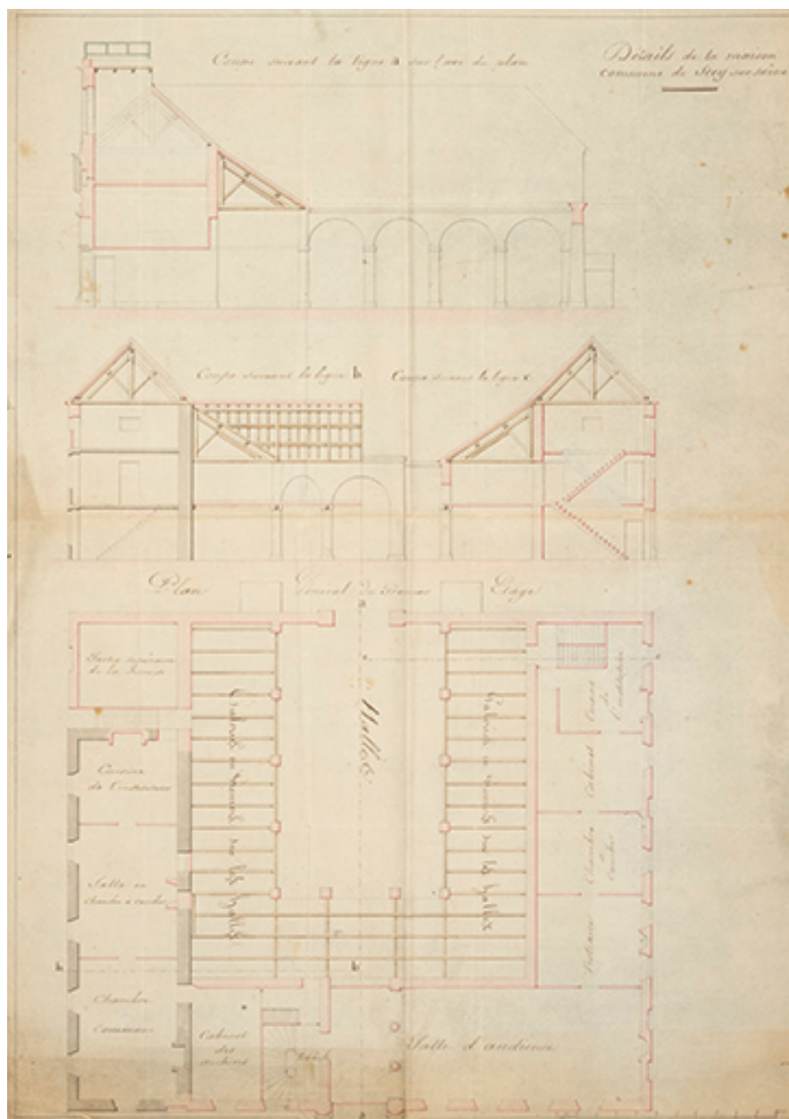
Détails de la maison commune de Scey-sur-Saône. Coupe. Plan général du premier étage. [1831].
