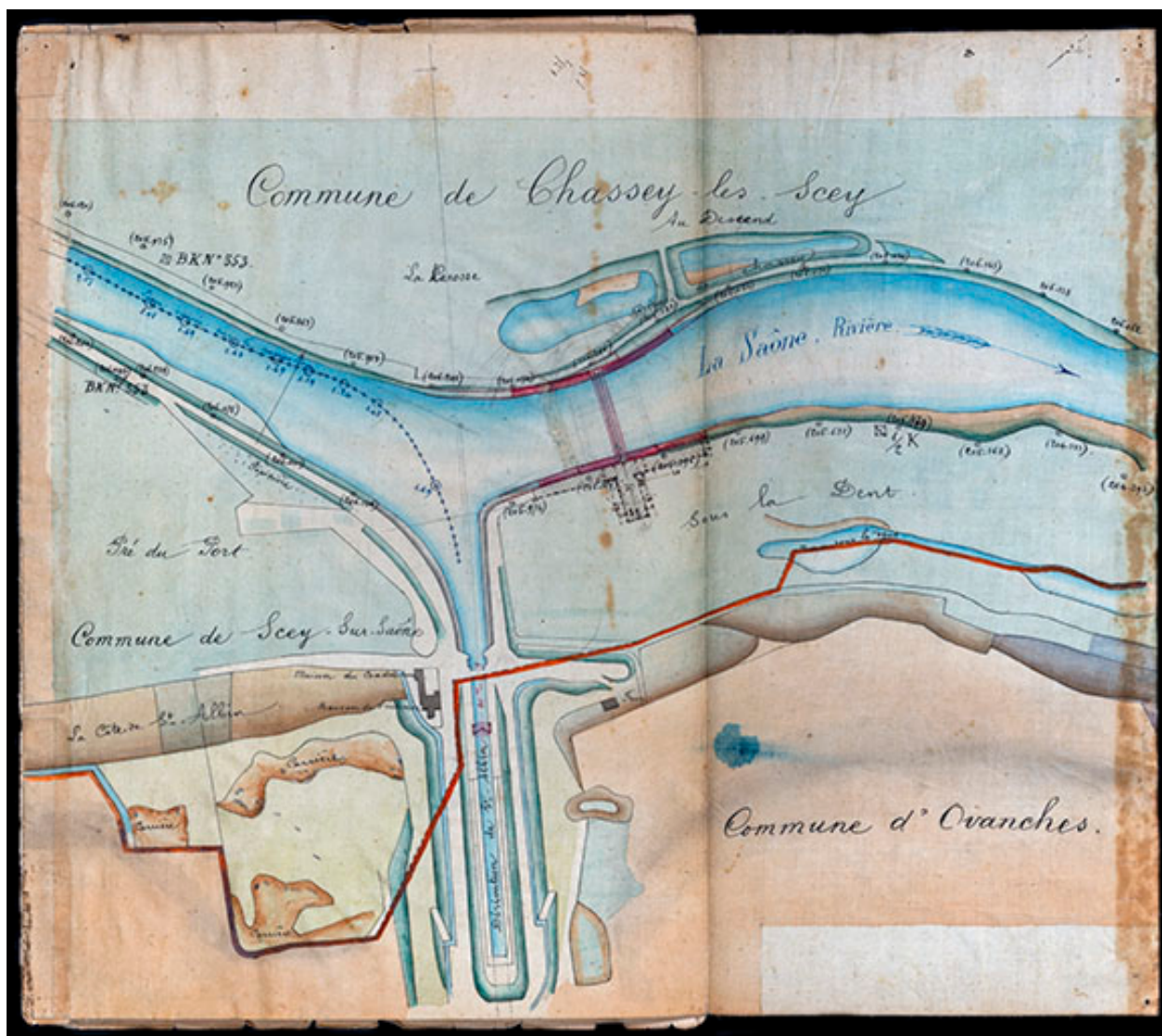
Construction du barrage mobile et de la seconde porte de garde de St-Albin - Plan des abords du barrage (1876).
