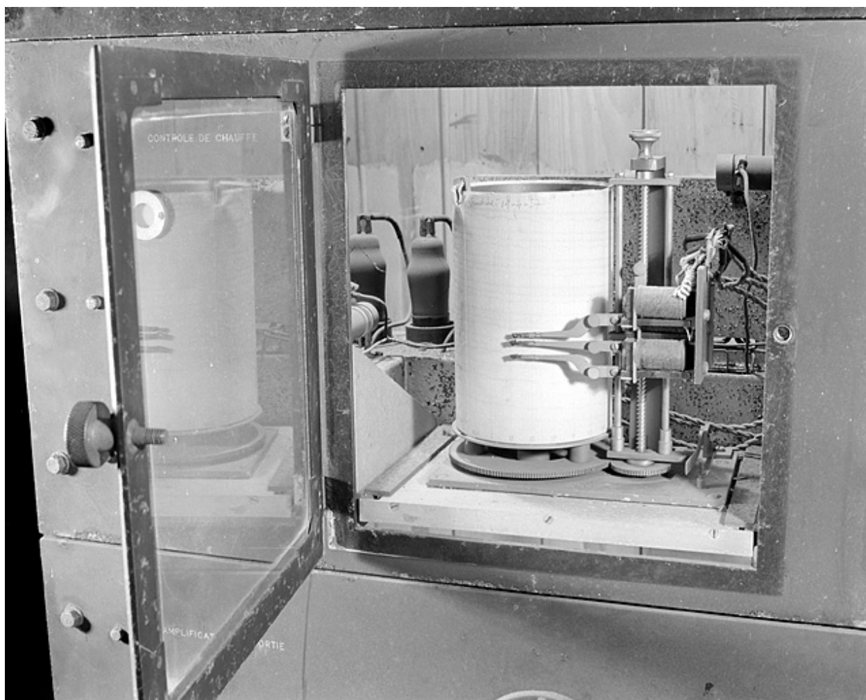
Diapason étalon : dispositif d'enregistrement de la température.
