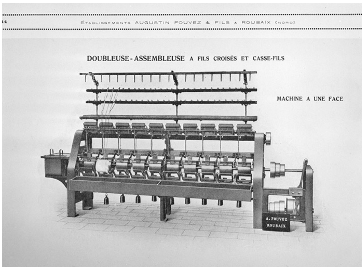
Doubleuse-assembleuse à fils croisés et casse-fils.
