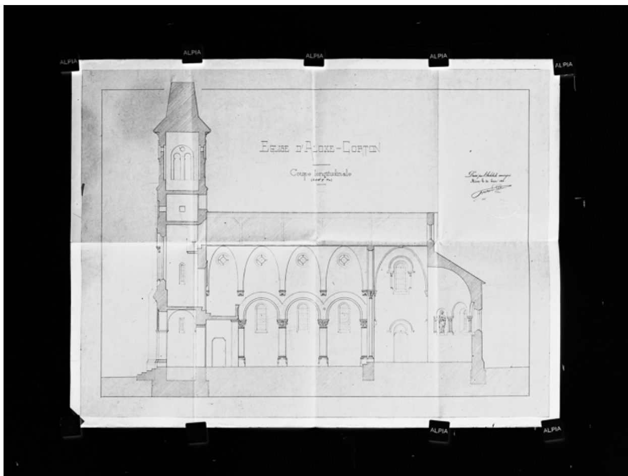
Coupe longitudinale de l'église d'Aloxé-Corton, dressée par l'architecte Pinchard le 30 juin 1888 (Archives communales, Aloxé-Corton).
