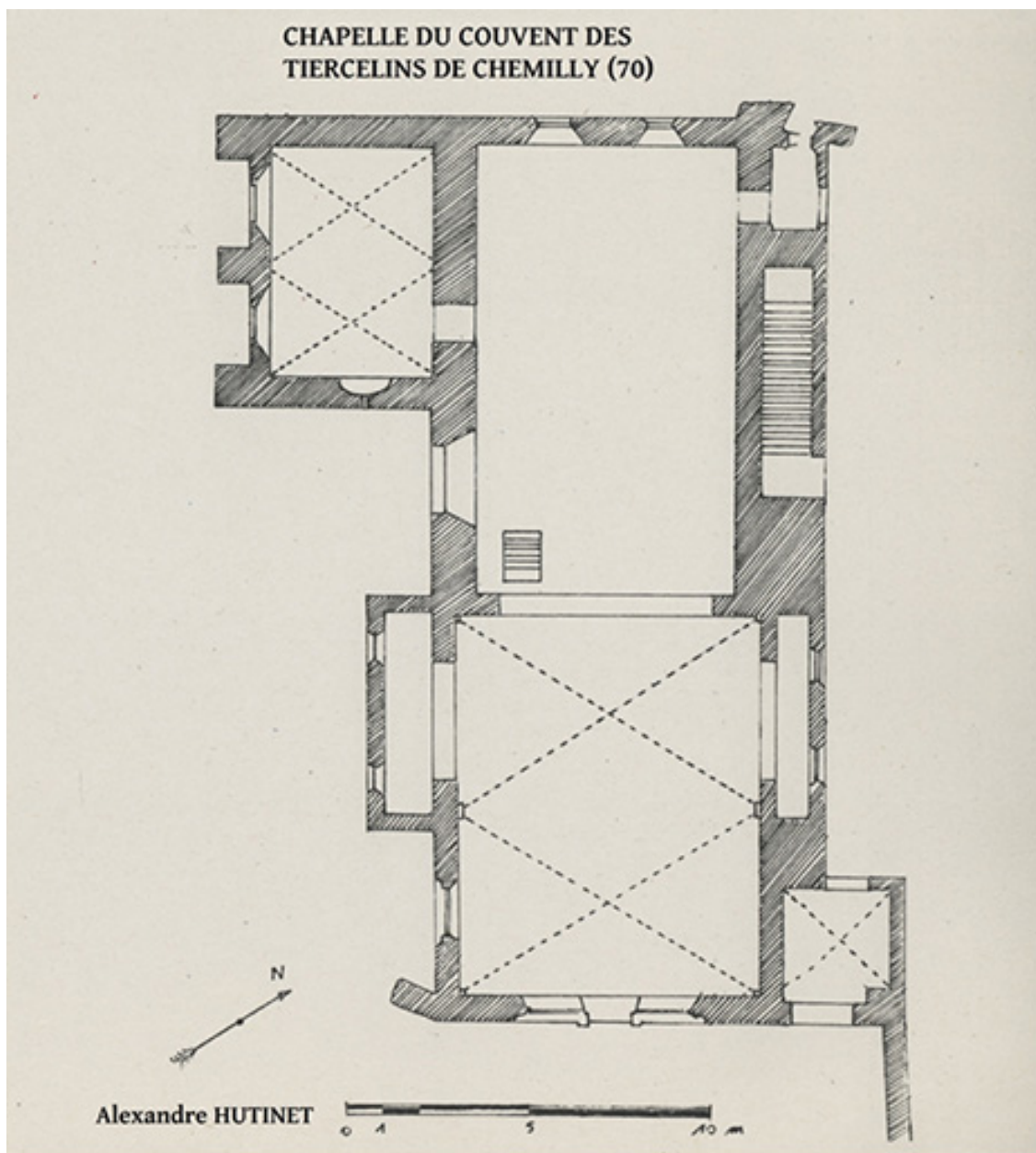
Plan de la chapelle du couvent de Chemilly
