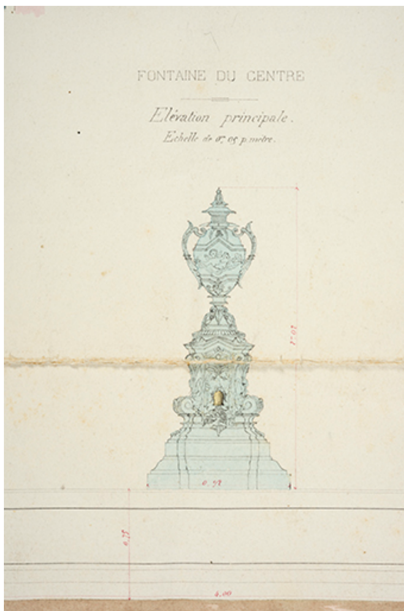
Fontaine du centre. Élévation principale. [Détail du plan] 1867
