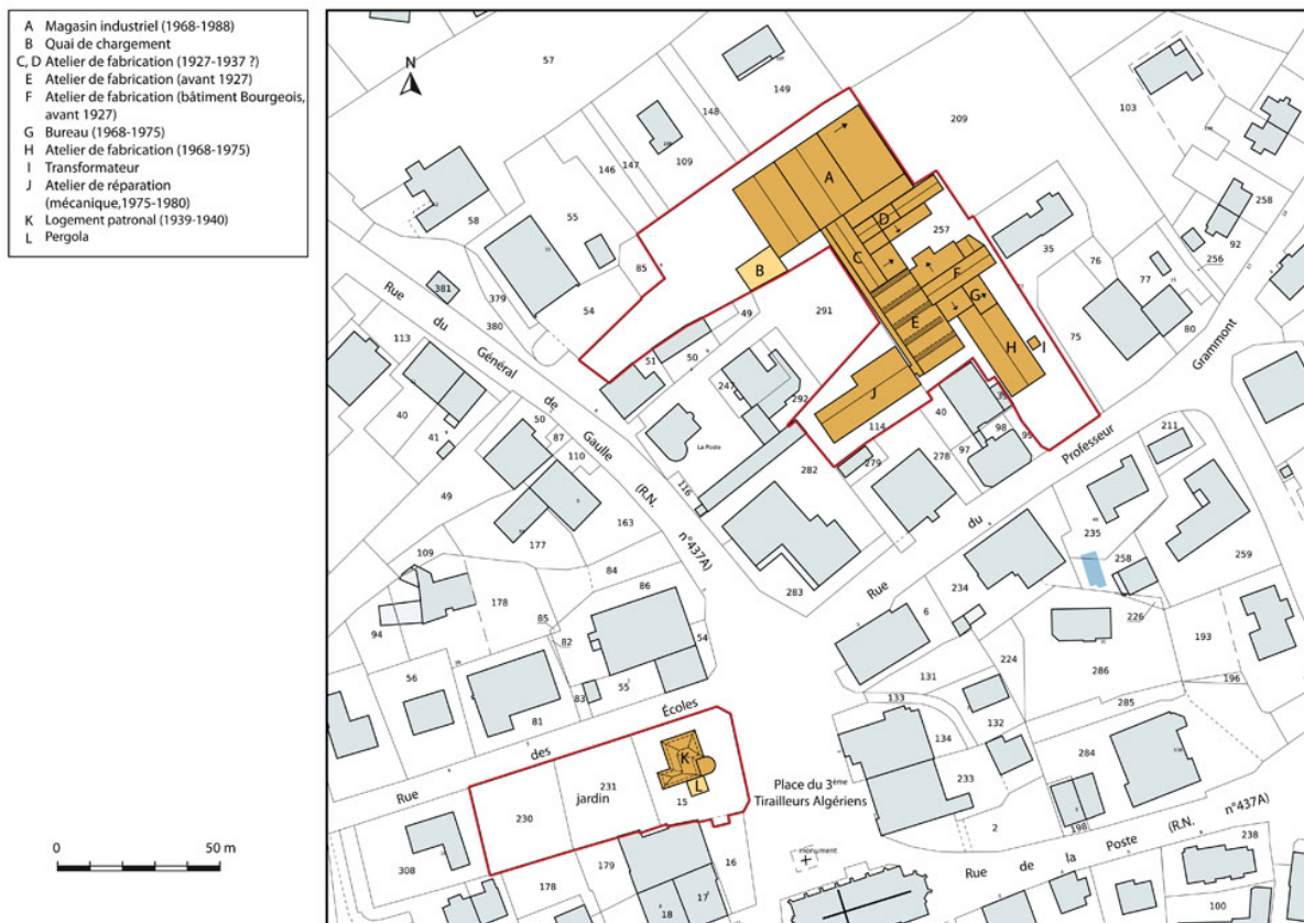
Plan-masse et de situation. Extrait du plan cadastral, 2012, sections AC et AE.
