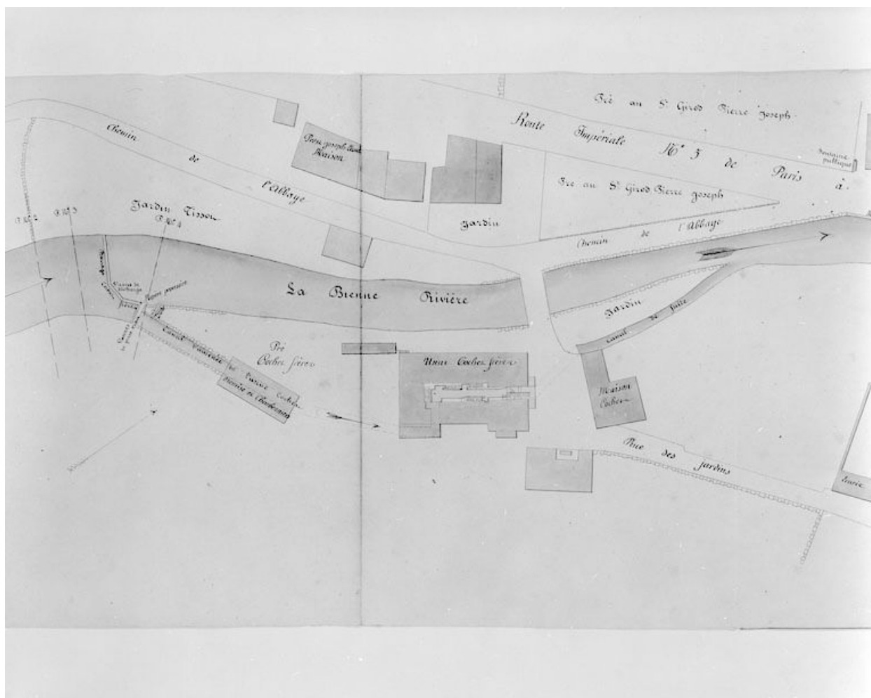
Réglementation de l'usine des s.s. Cochet frères. Plan des lieux et dessins de détail. Dessin, 1863. Echelle 1:500.
