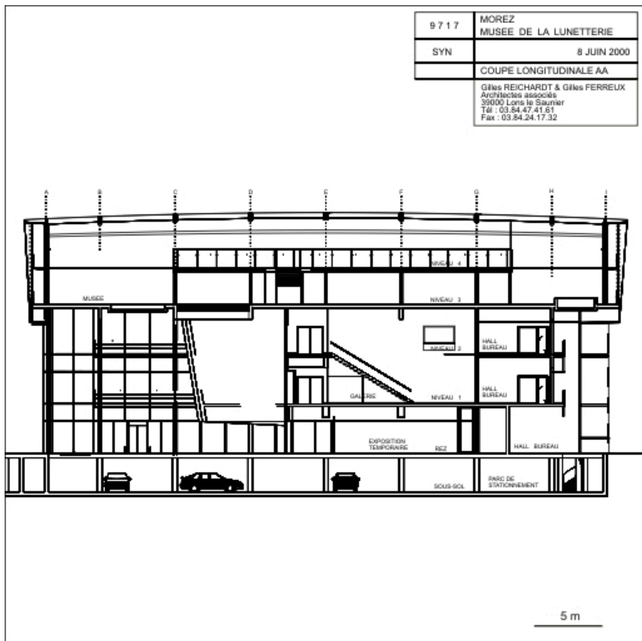
Coupe longitudinale AA, 2000.
