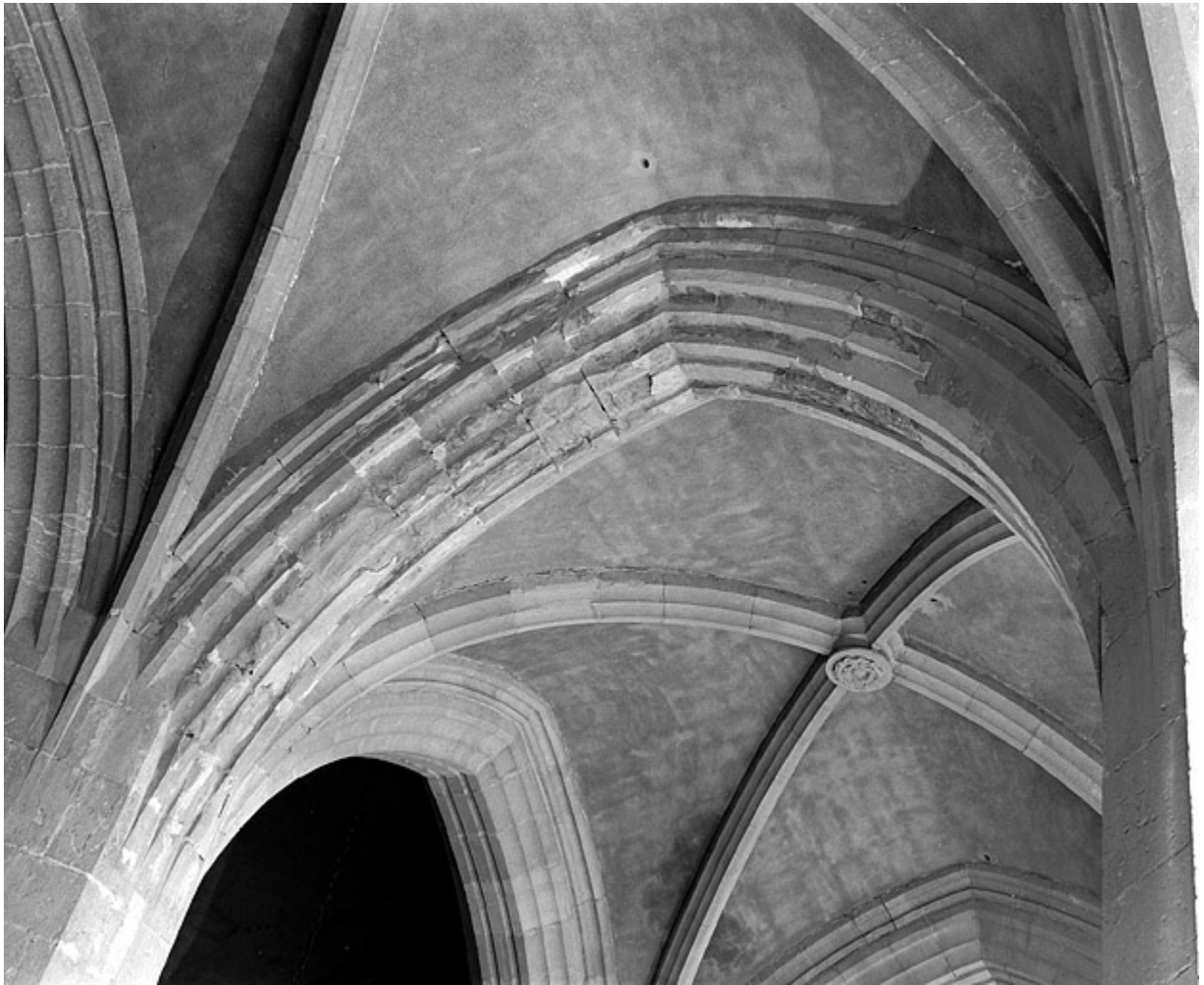
Doubleau entre les quatrième et cinquième travées du collatéral sud.
