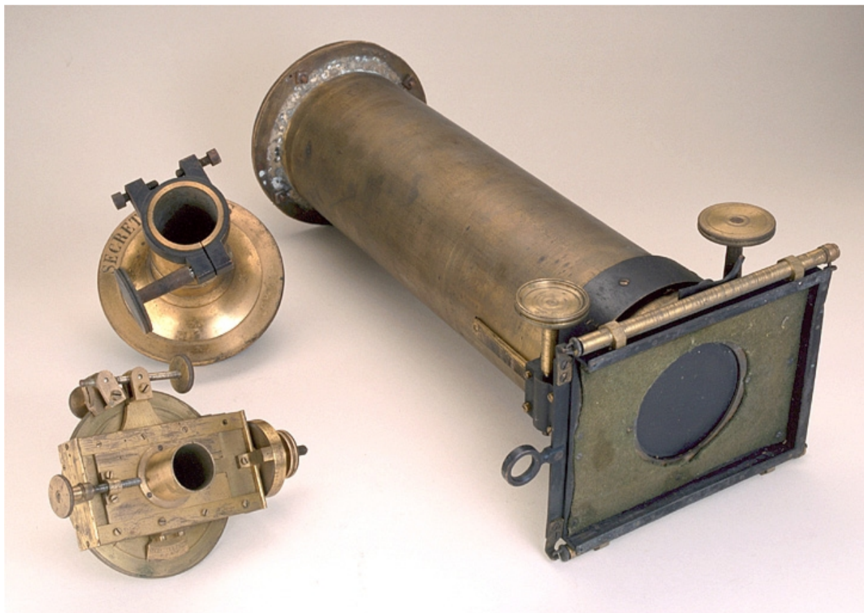
Vue d'ensemble du tube avec porte-plaque à crémaillère (à droite), accompagné du micromètre (au 1er plan) et du porte-oculaire (au 2e plan).
