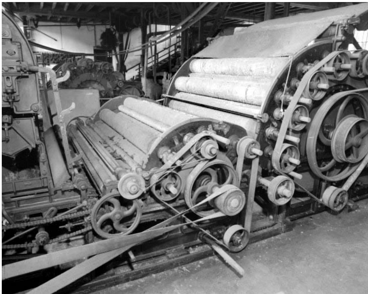
Cylindre briseur et avant-train.
