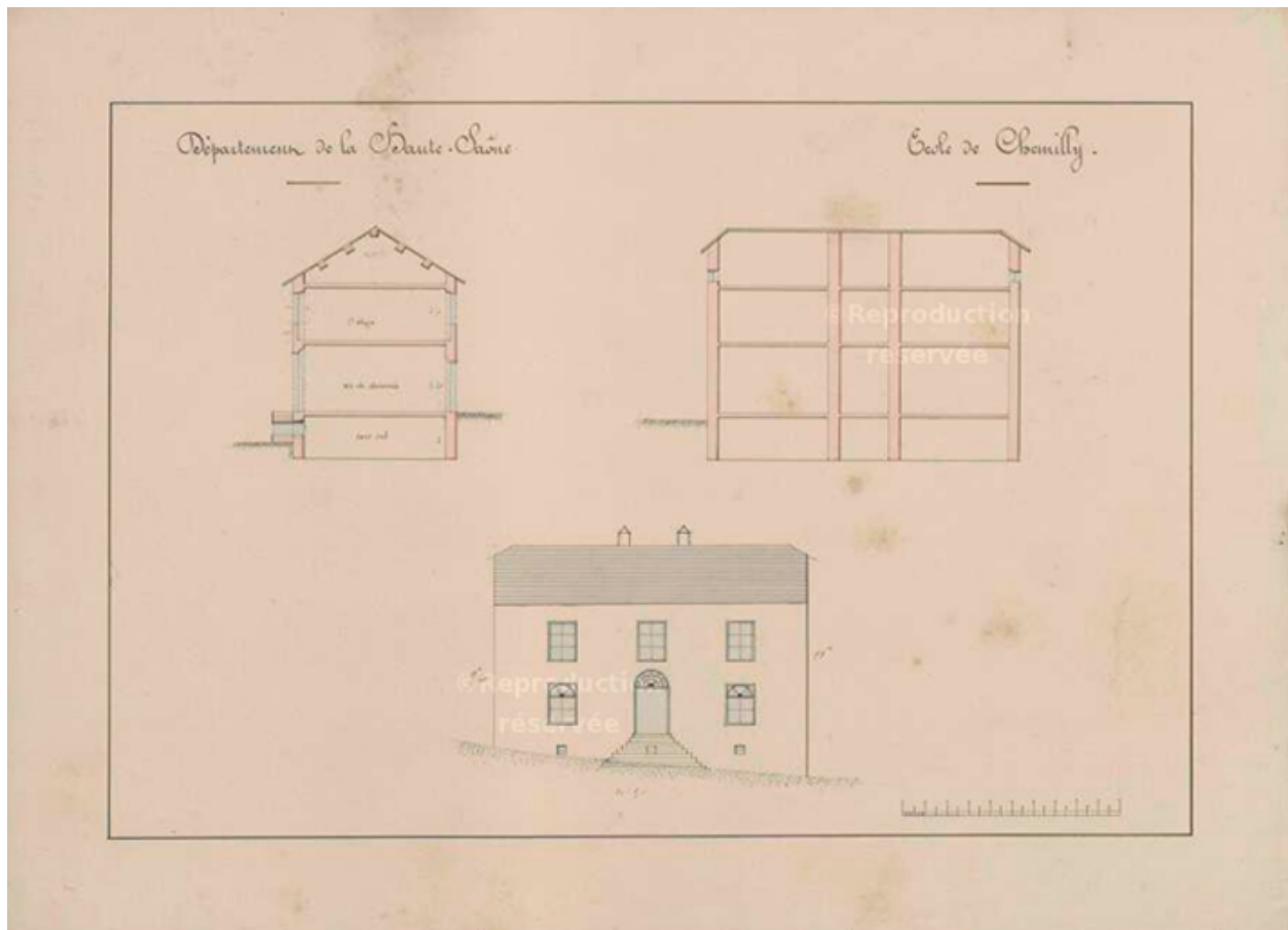
Plans en coupe et en élévation de la façade sur la rue de l'école de Chemilly
