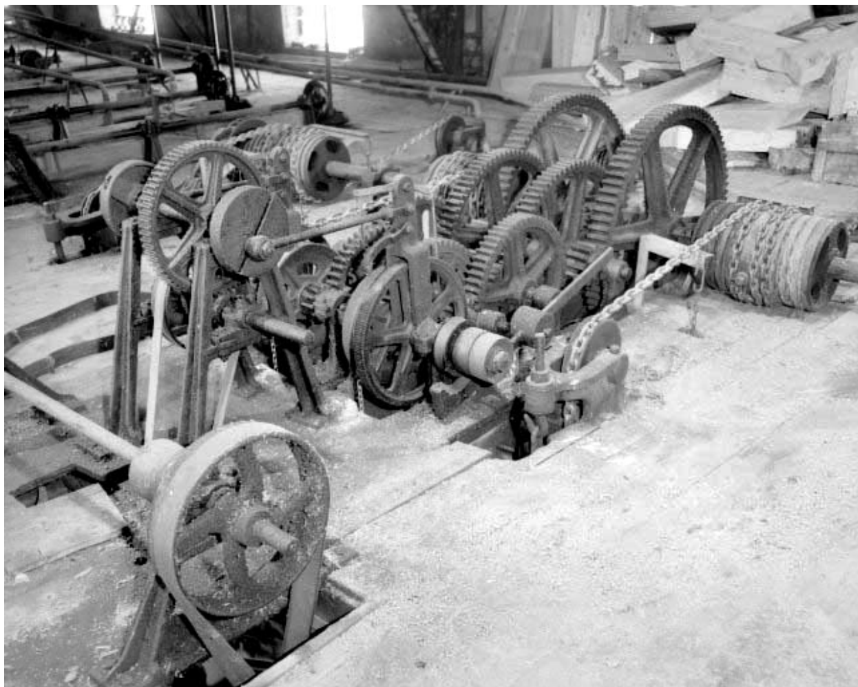
Système de descente à chaînes : détail.
