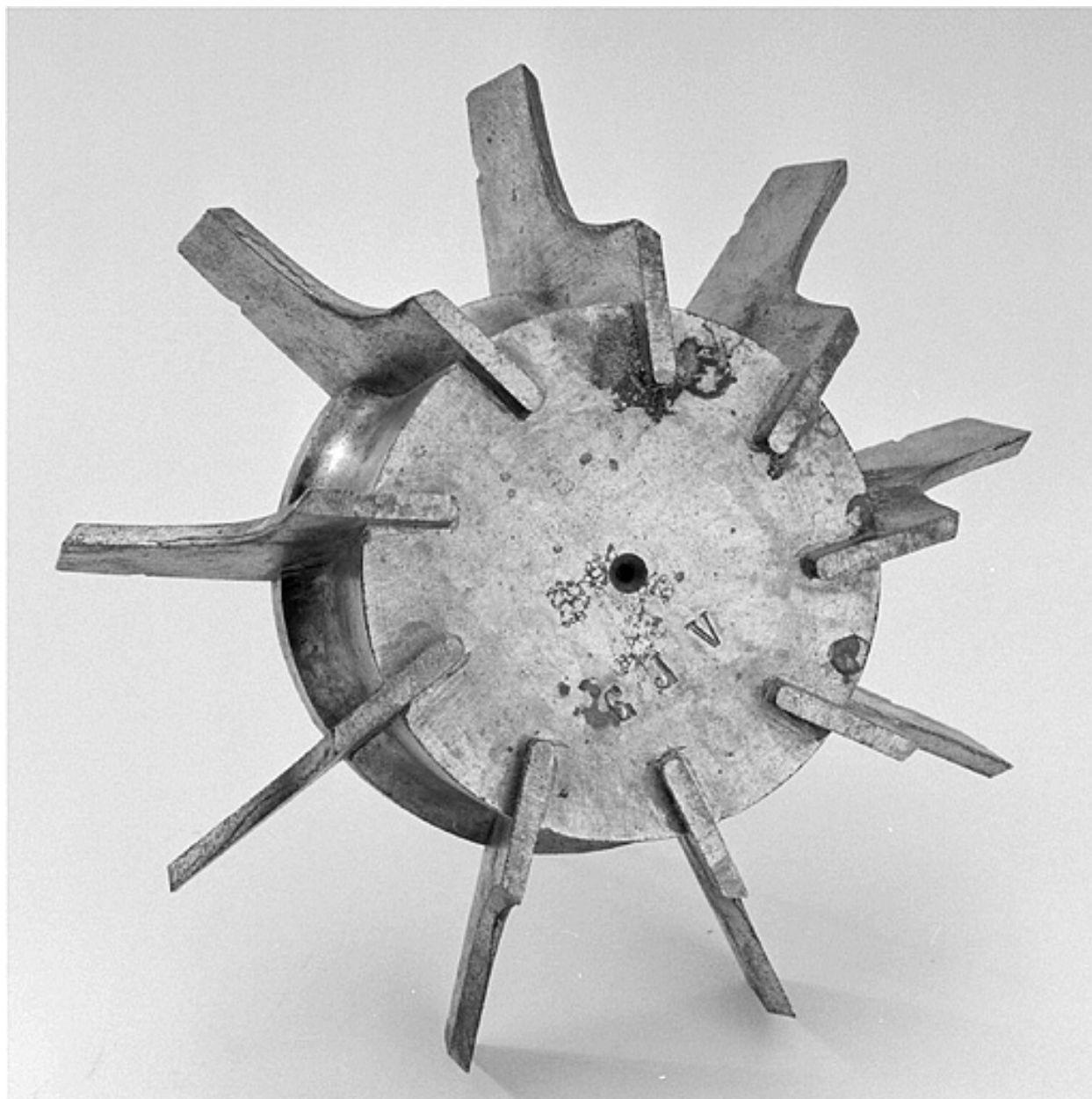
Détail d'une fraise vue de dessus.
