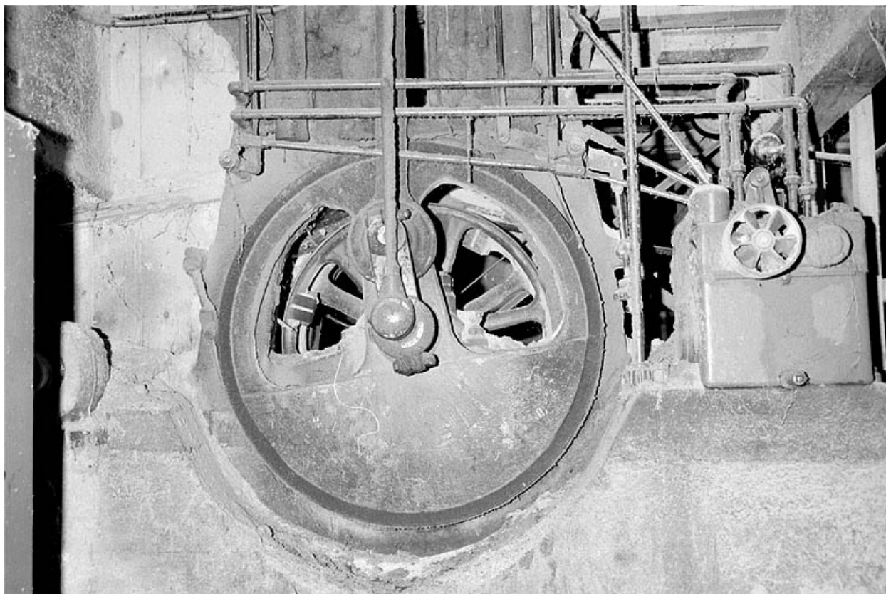
Usine de tournerie et scierie Janier-Vuillermoz, Lavans-lès-Saint-Claude (2-4 rue du Caton) : système d'entraînement du châssis de scie multilame Socolest.
