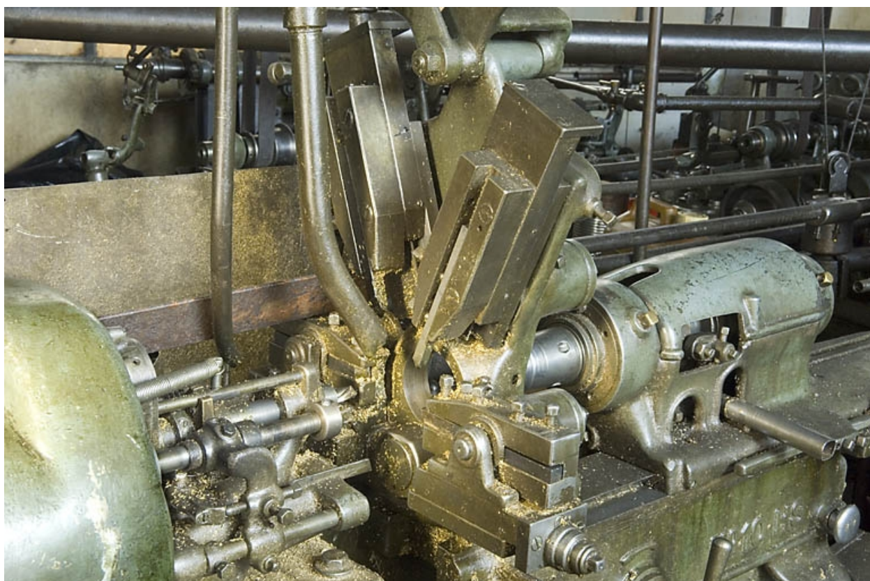
Tour à décolleter 10 HS Jos. Petermann (K). Détail.
