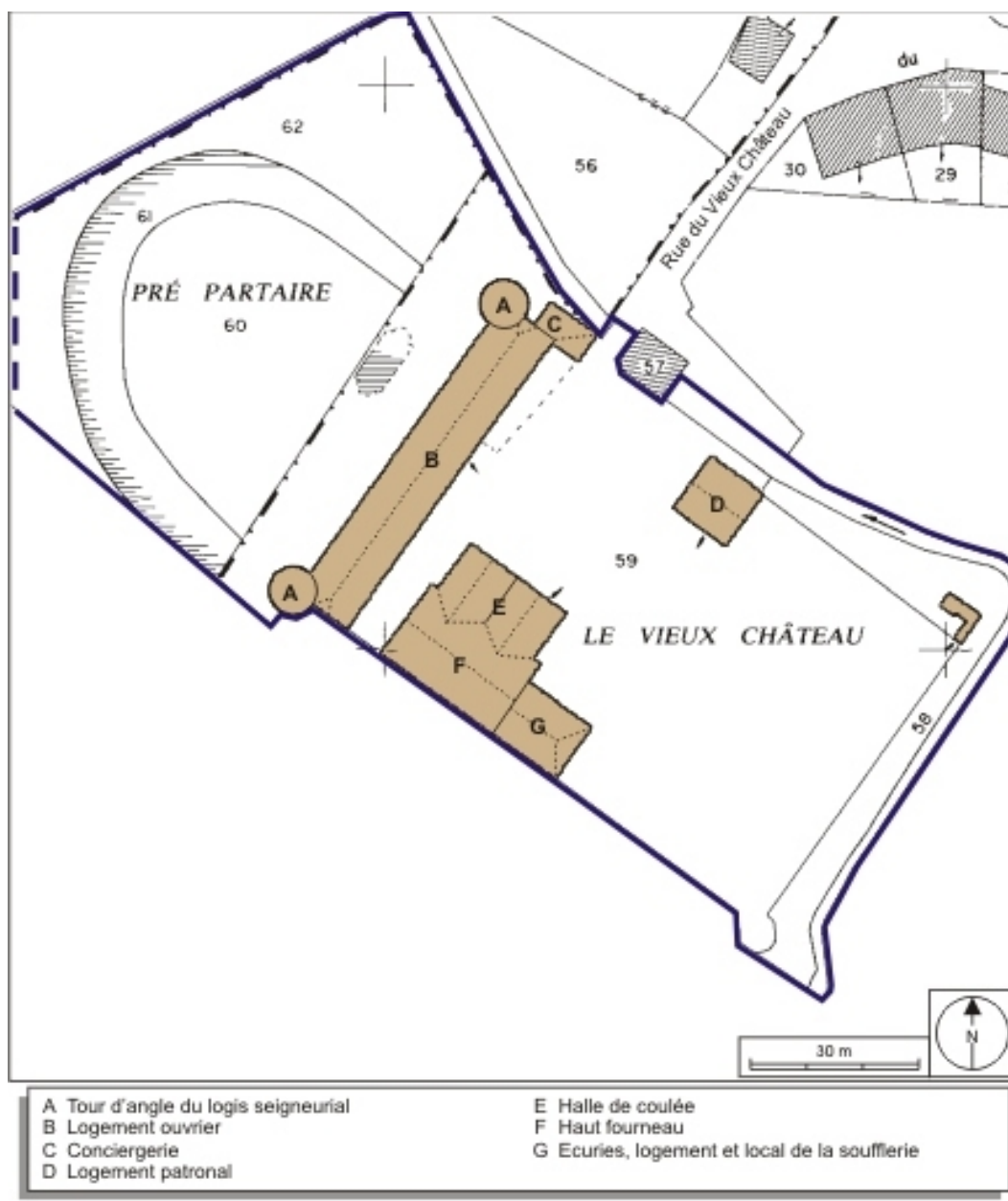
Plan-masse et de situation. Extrait du plan cadastral numérisé, 2008, section AC, 1:1000. Source : Direction générale des Finances Publiques - Cadastre ; mise à jour : 2008.
