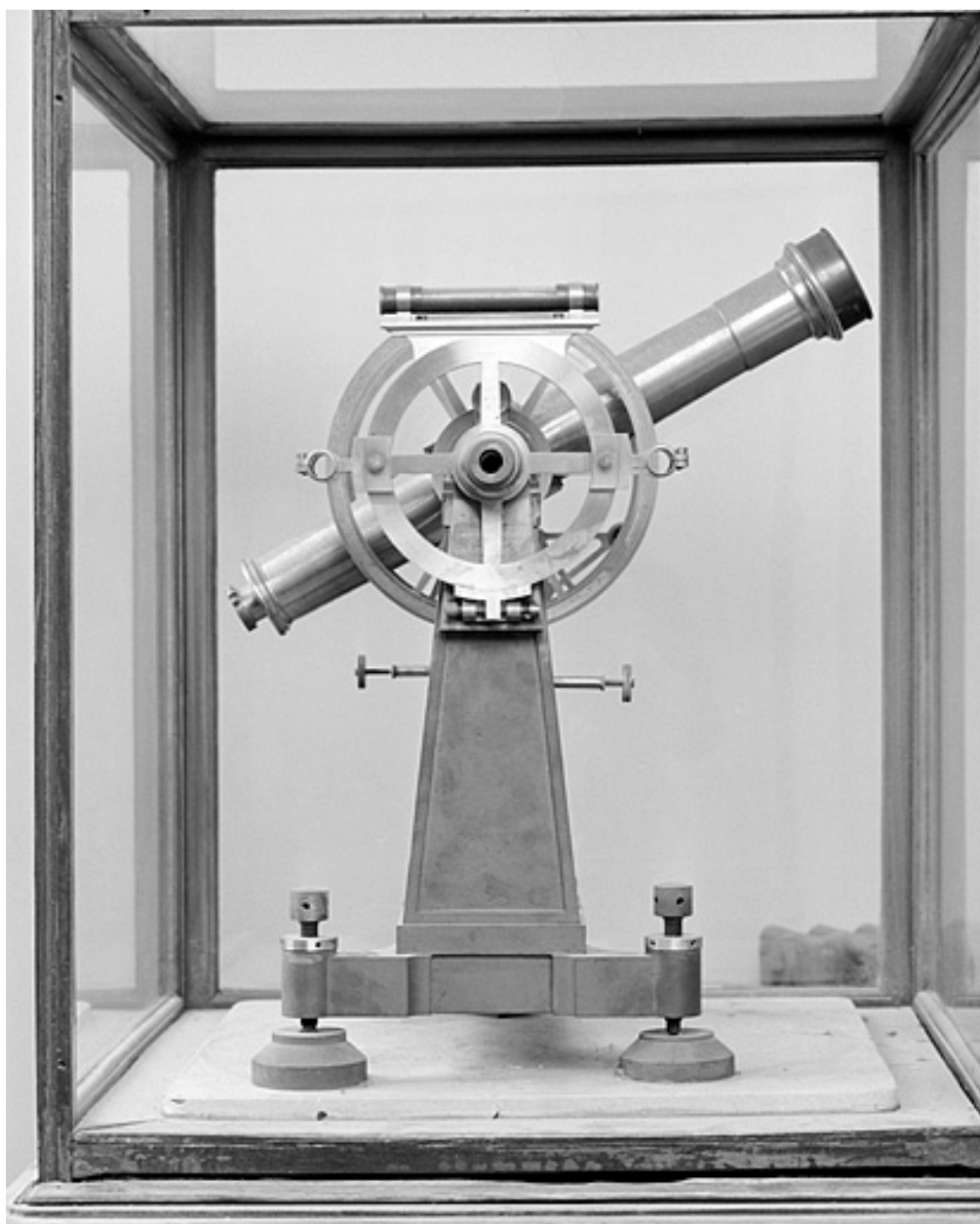
Profil, côté droit.
