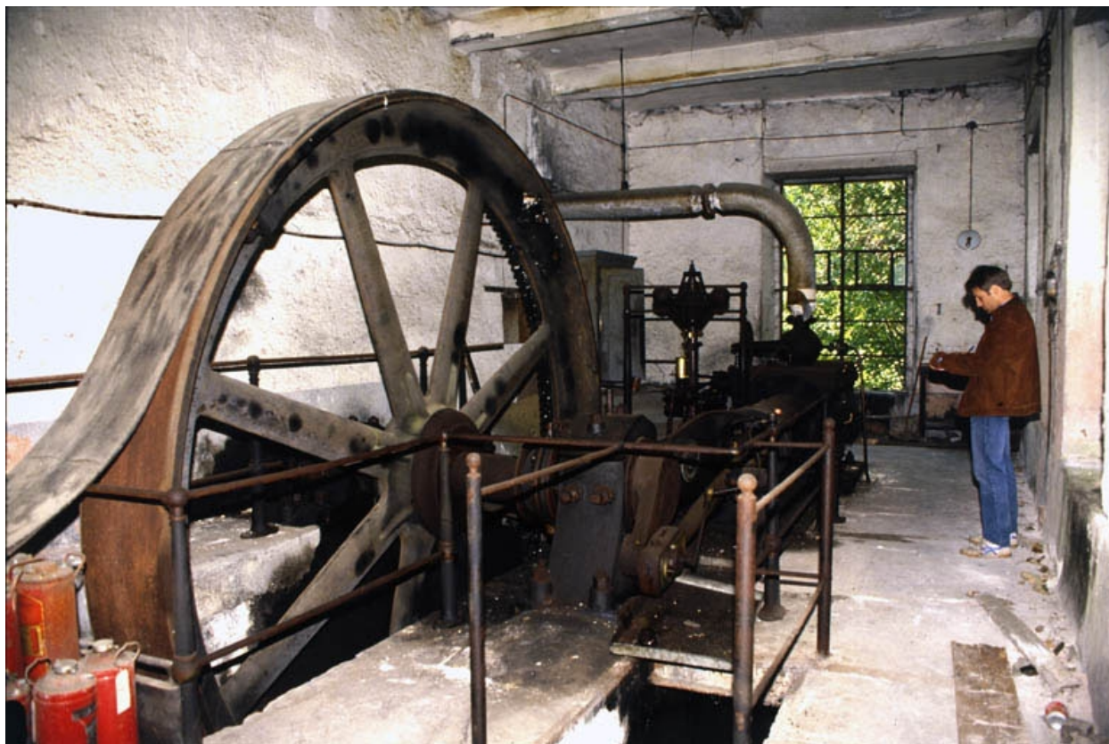
Vue d'ensemble de la salle des machines avec sa machine à vapeur.
