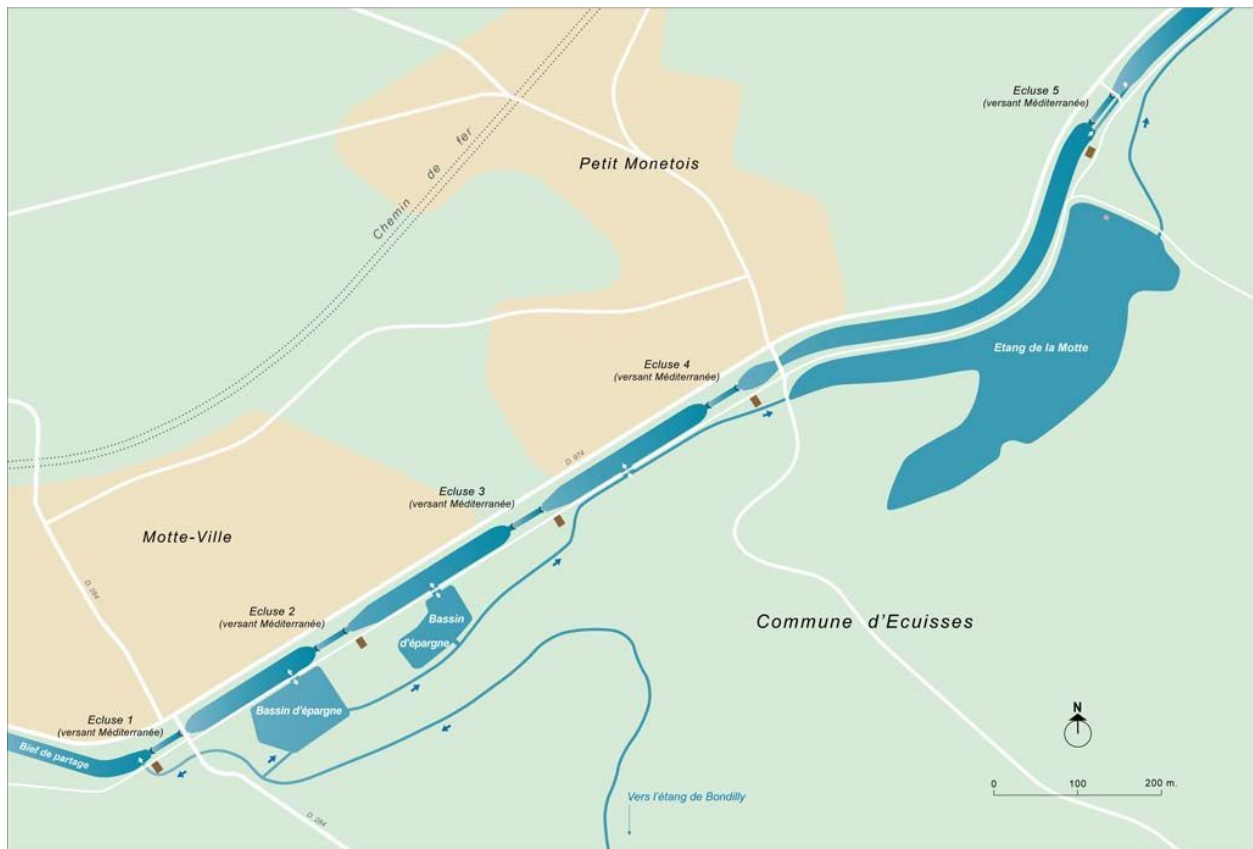
Carte schématique de l'alimentation de l'échelle d'écluses d'Ecuisses.
