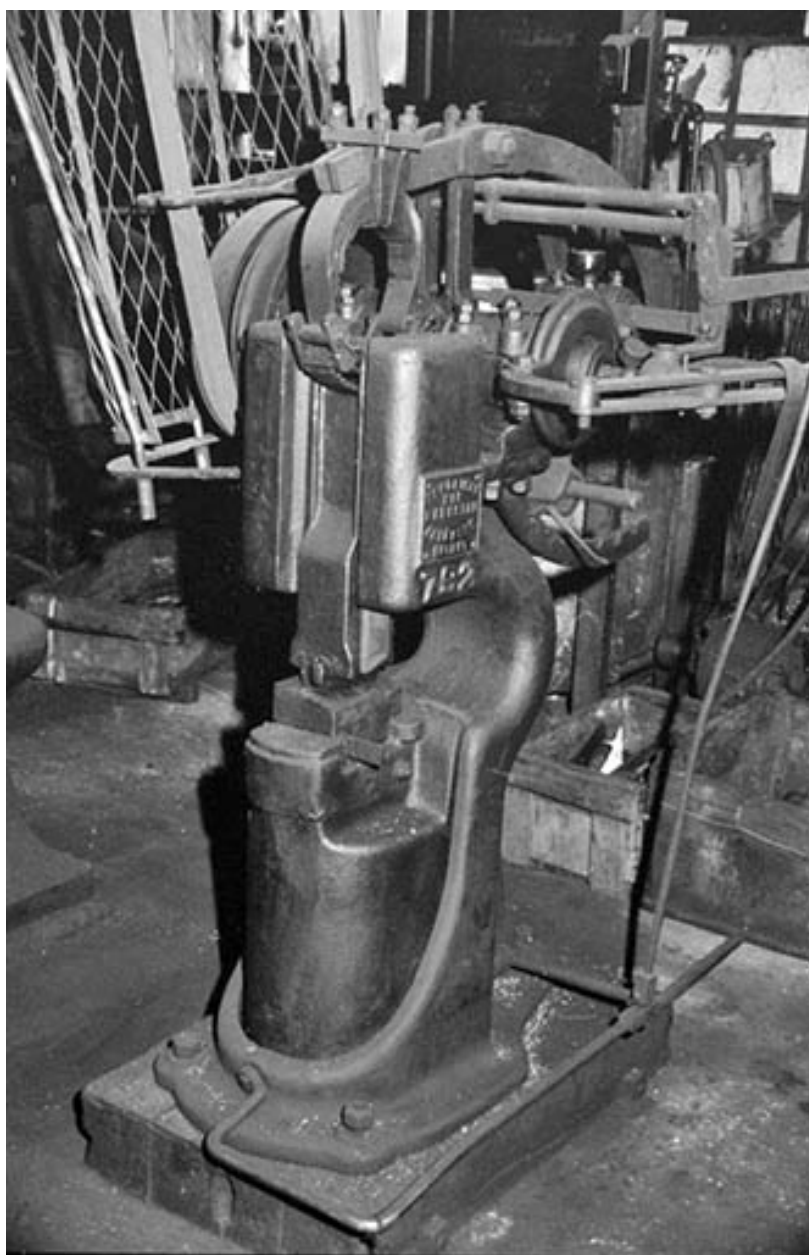
Marteau-pilon : détail. Plaque : Enköpings . Mek . Verkstad . Enköping . Patent . 792.
