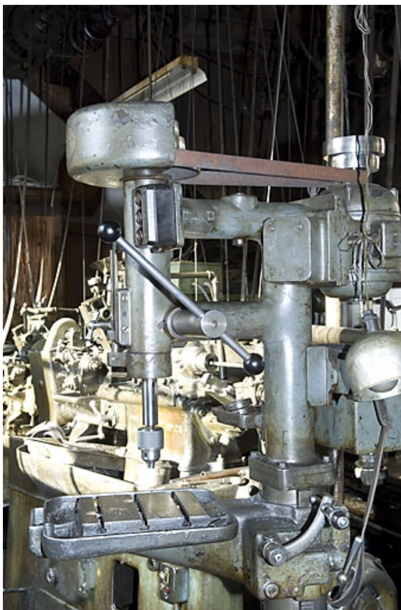
Perceuse à colonne (I).
