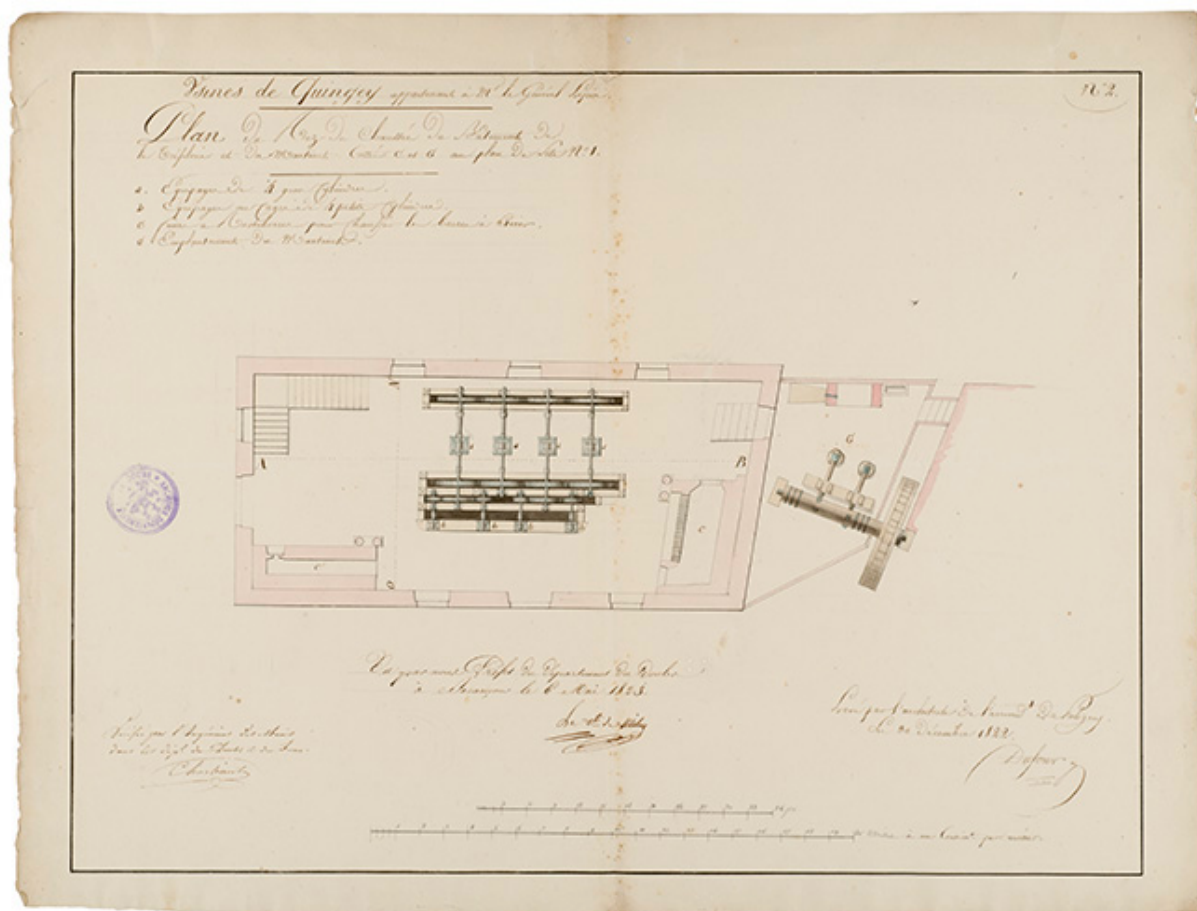
Usines de Quingey [...]. Plan du rez-de-chaussée du bâtiment de la tréfilerie et du martinet [...], 1822.
