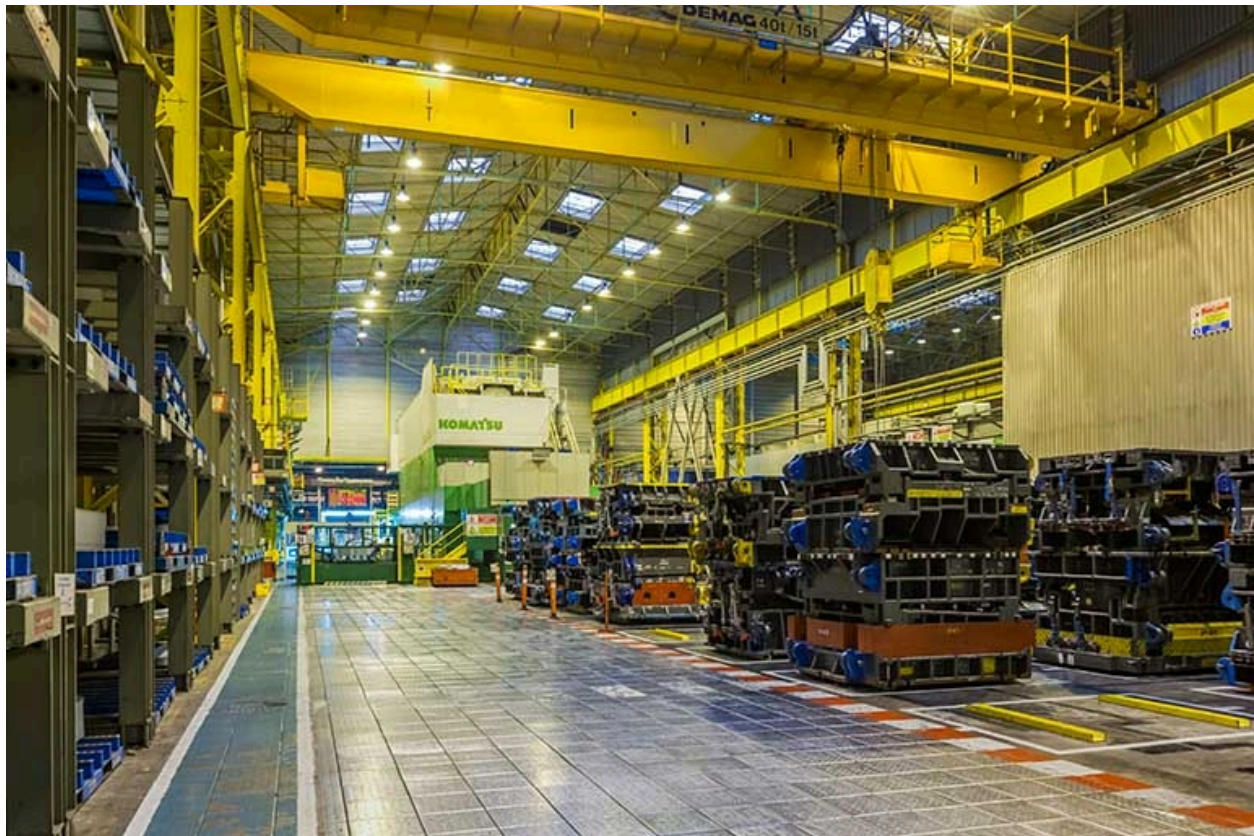
Atelier d'emboutissage. Presse Komatsu et outils de presses (matrices) au premier plan.
