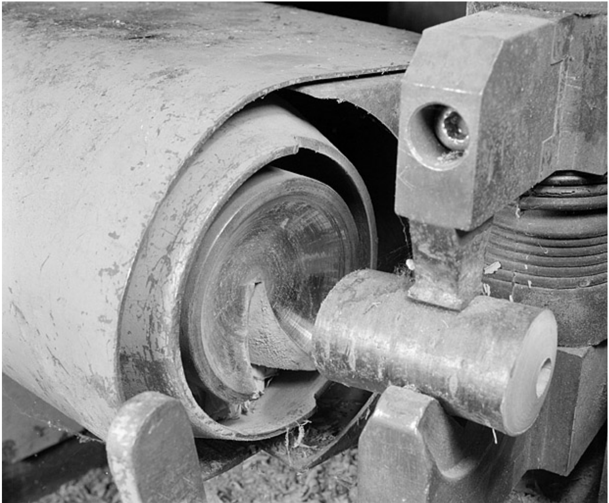
Détail de l'outil de coupe côté gauche.
