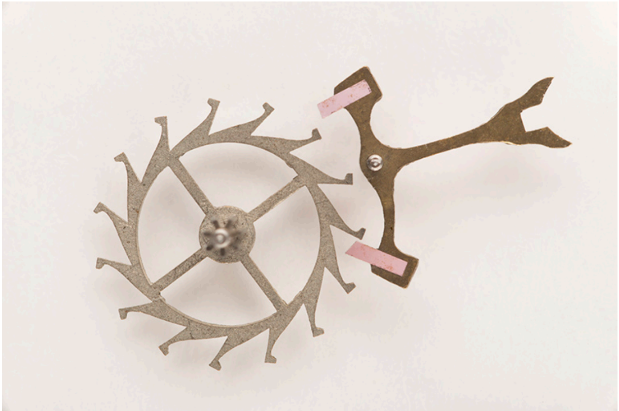
Echappement à ancre.
