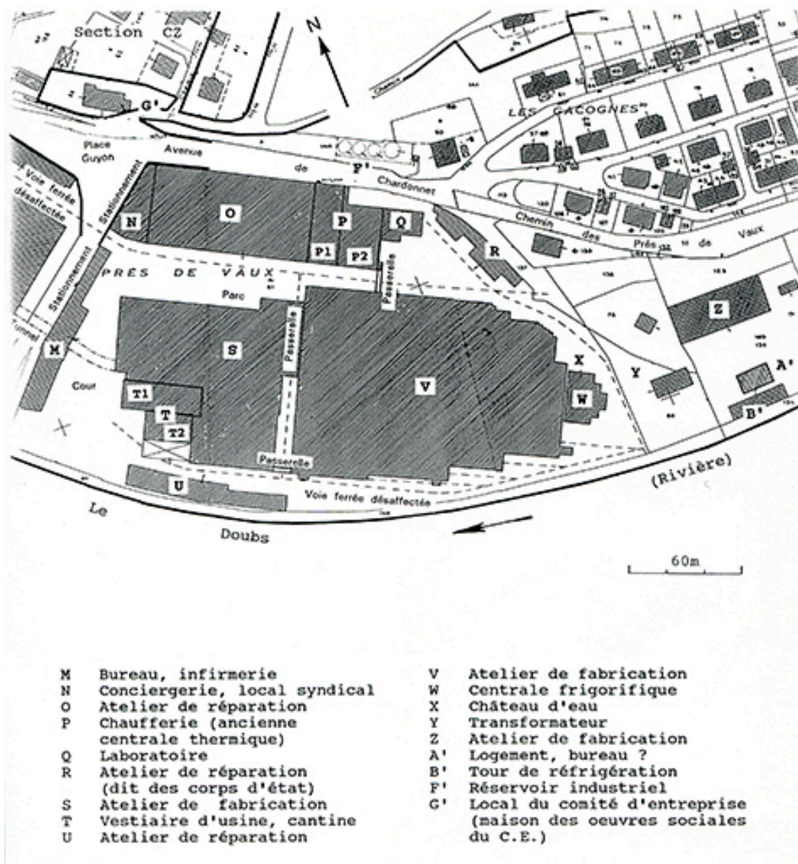
Plan-masse de la partie centrale du site industriel (usine A). Extrait du plan cadastral, 1982, section DH, 1/1 000 réduit à 1/2 000.
