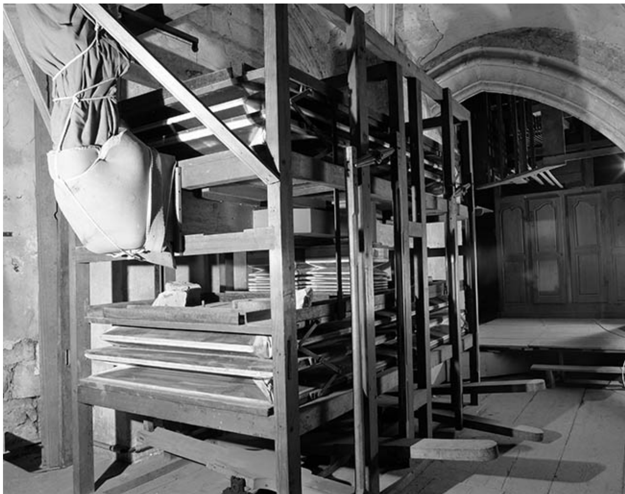
Soufflerie, vue de trois quarts gauche.
