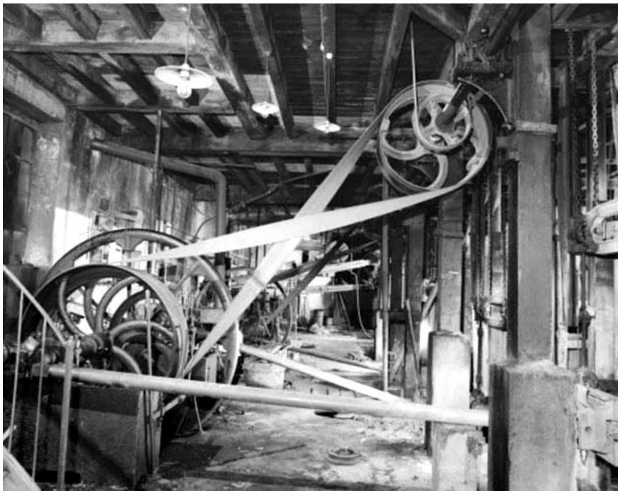
Transmission des châssis multilames.
