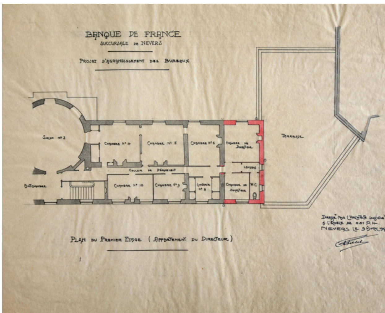
Plan du premier étage, projet d'extension (9 avril 1907).
