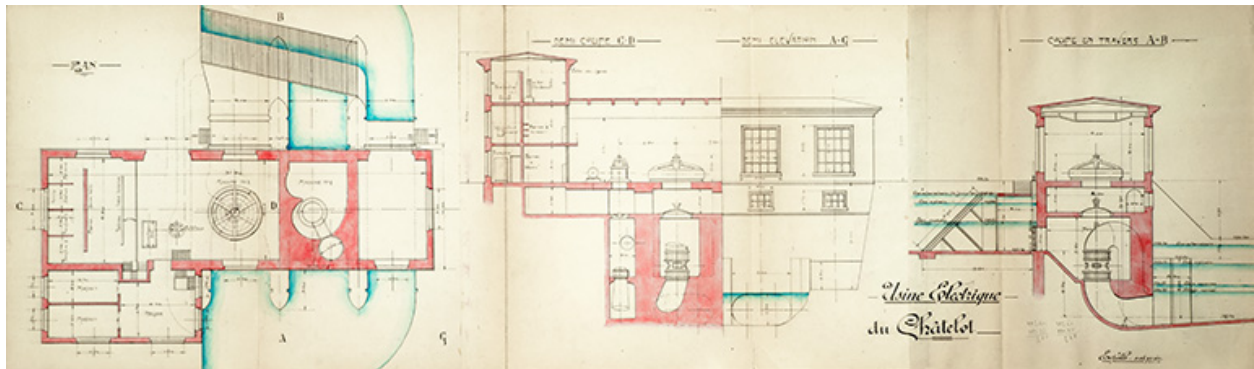
Usine électrique du Châtelot, plan, coupe, élévation, 1917.
