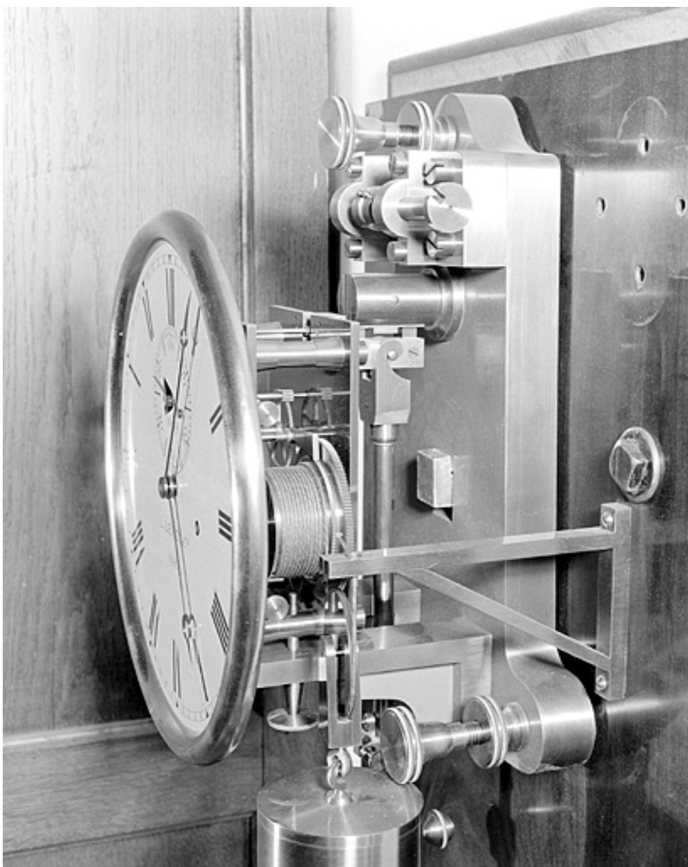
Cadran et mécanisme, vus de profil.
