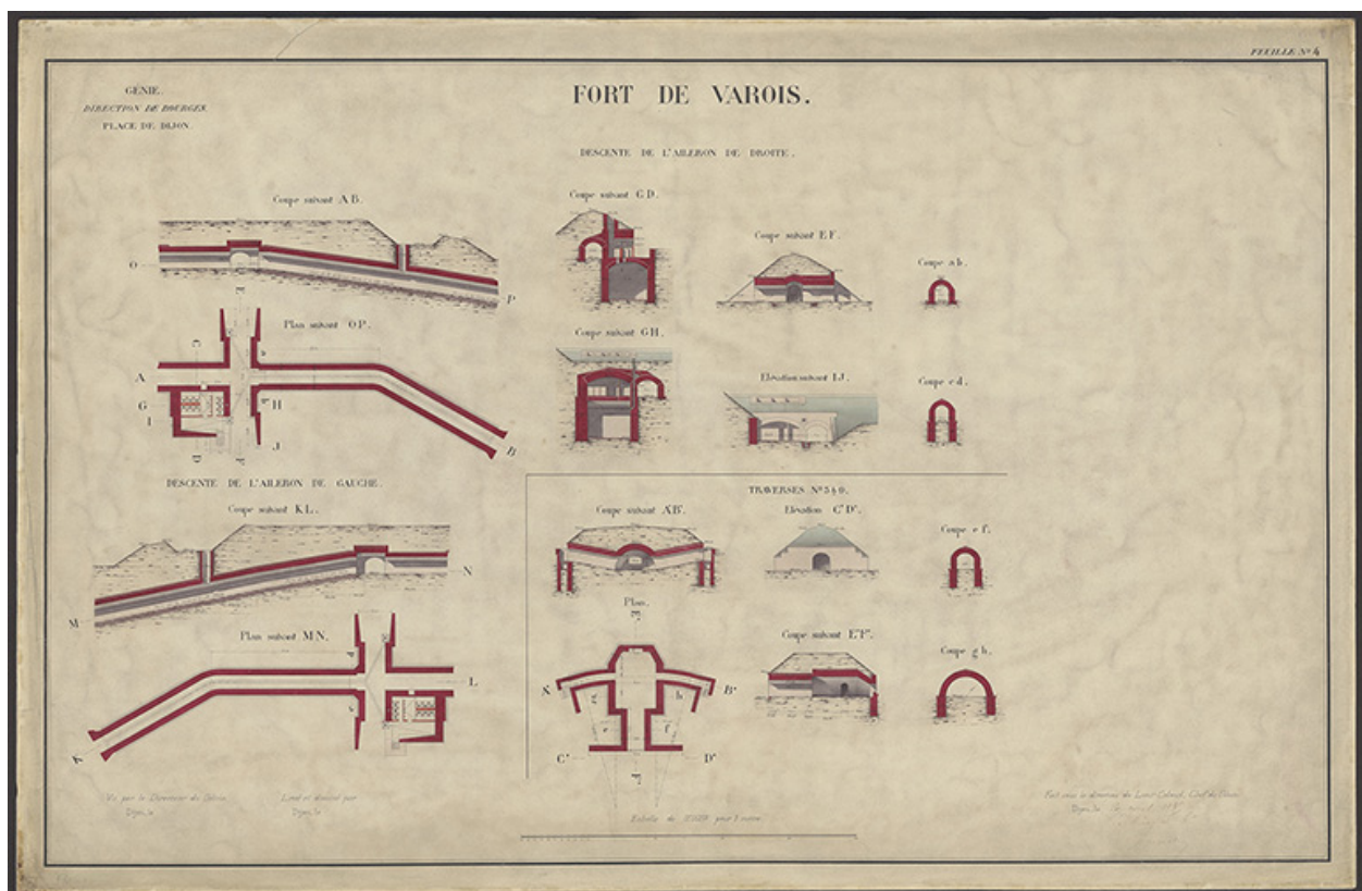
Fort de Varois. Descente de l'aileron de droite. 1885.
