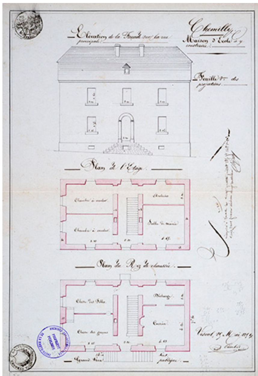
Plans de la façade sur rue de l'école à construire, 1851
