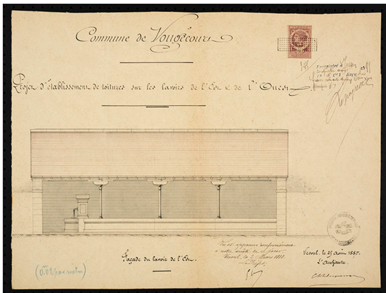
Projet d'établissement de toitures sur les lavoirs de l'est et de l'ouest. [Élévation] 1887
