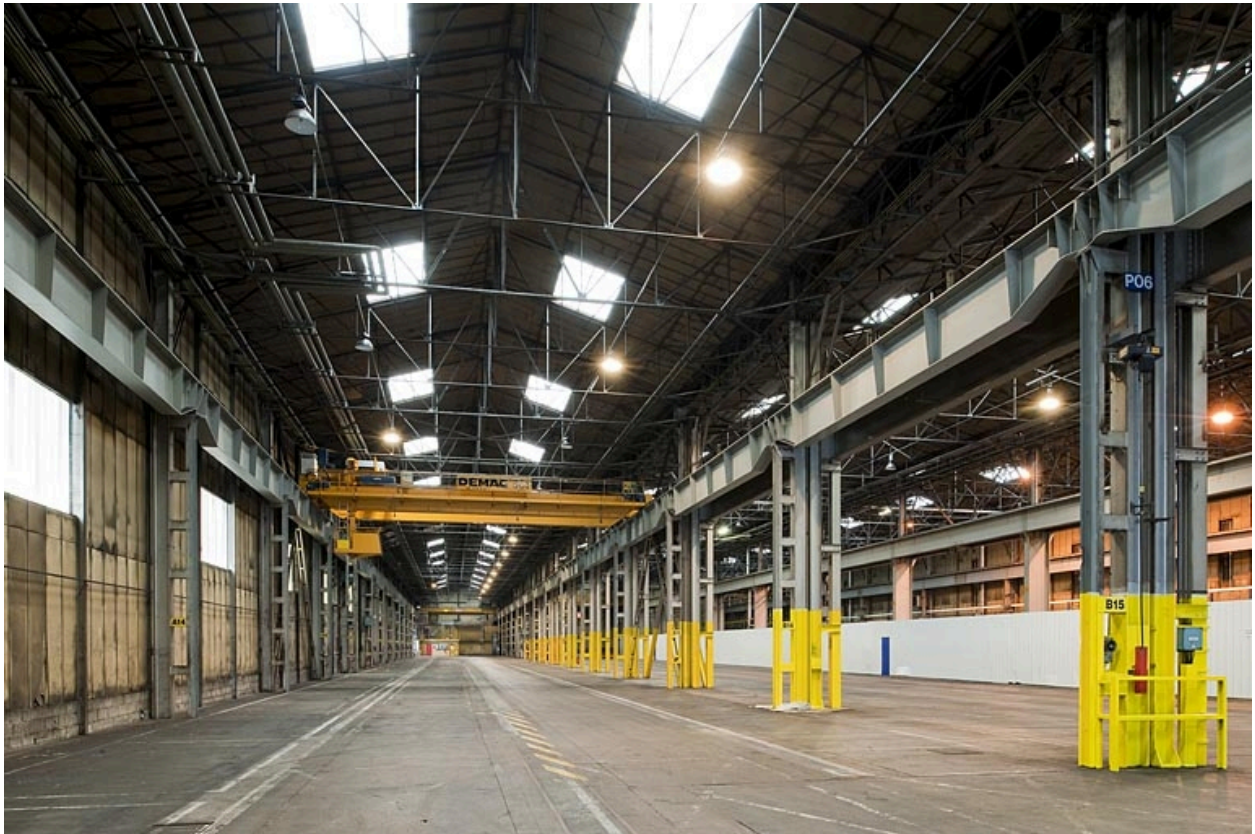
Halle métallique M 14. Vue axiale.
