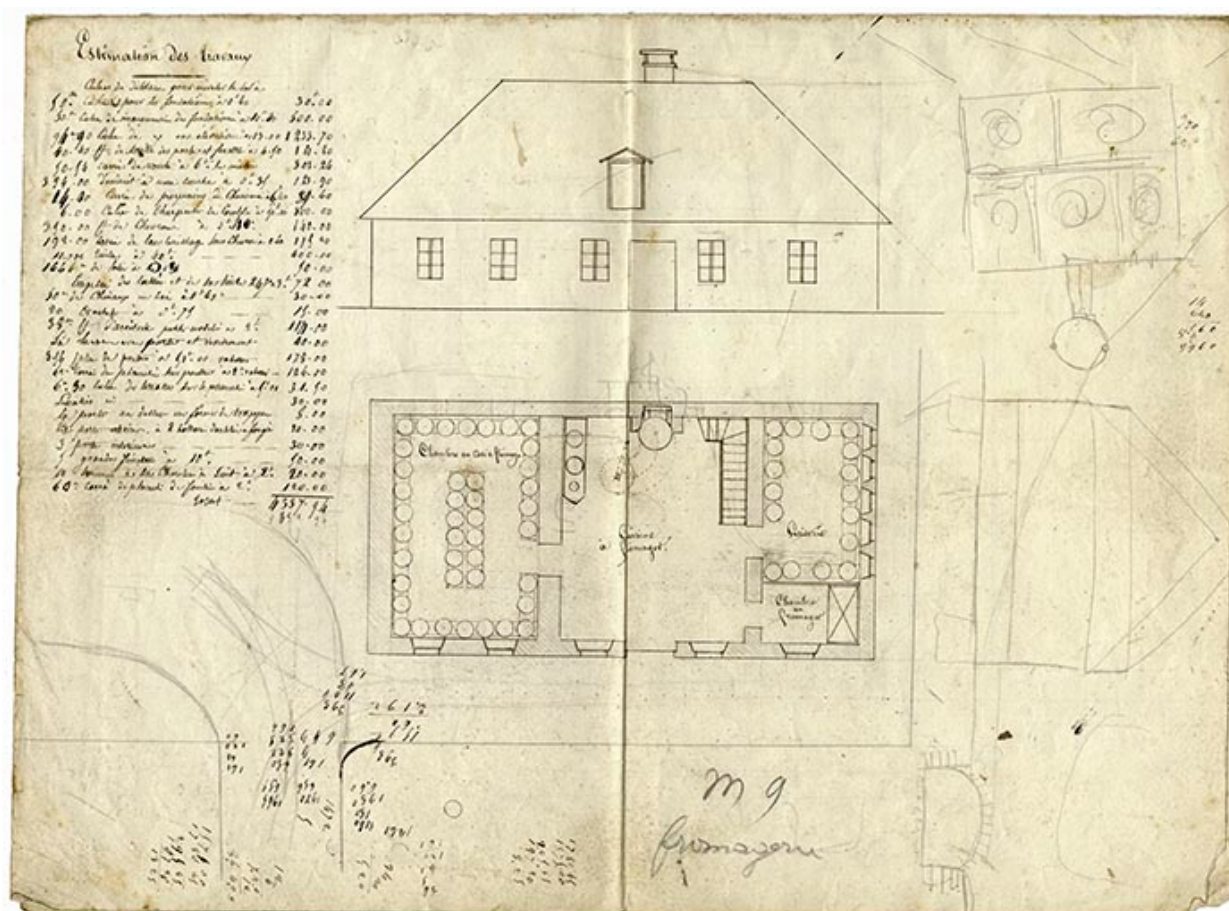
[Projet de fromagerie : plan et élévation], 1859.
