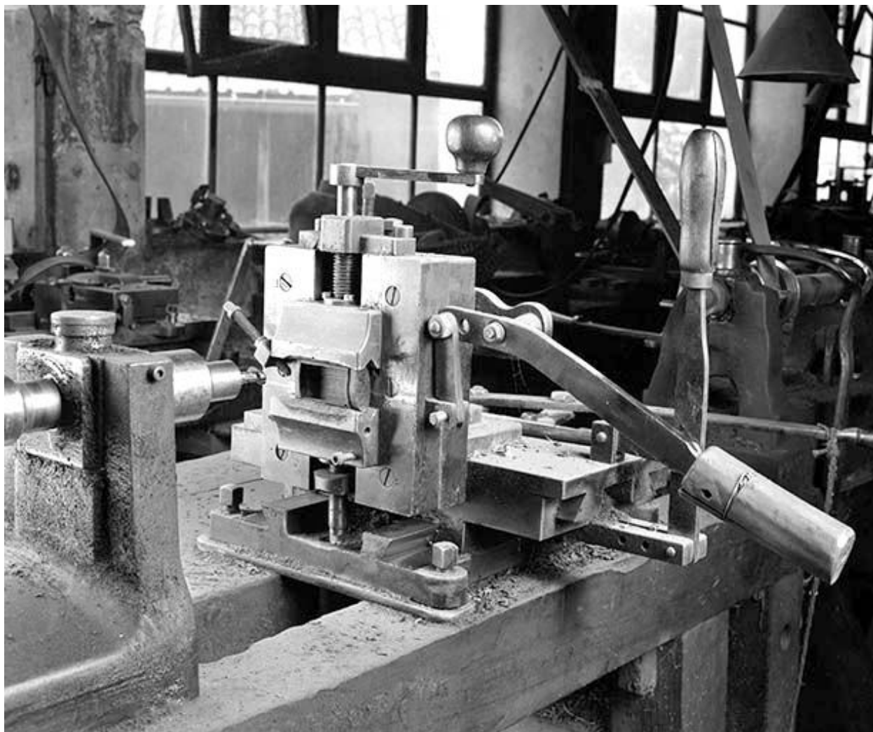
Usine de tabletterie (usine de pipes et de tabatières) Vincent-Genod, Saint-Claude (2 chemin de la Combe du Marais, 11 rue Carnot) : machine à fraiser (machine à renfoncer).
