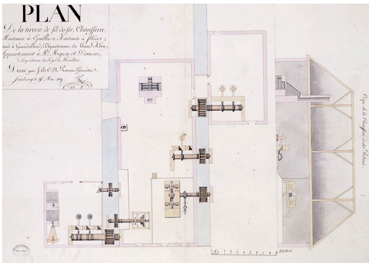
Plan de la tirerie de fil-de-fer, chaufferie, marteaux à épauler et martinets à filières [...] [coupe longitudinale et plan au sol].
