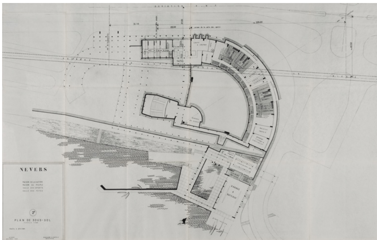
Nevers Centre municipal [...] 2B. Plan de sous-sol. Novembre 1960-mars 1961.
